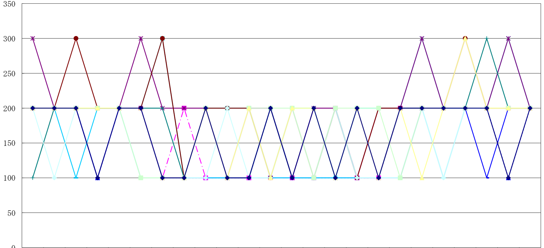
〔使用電力量kWh〕 各月指定日(最大電力量計測日)のロードカーブ(令和4年10月～令和5年9月)(石元受電所)
