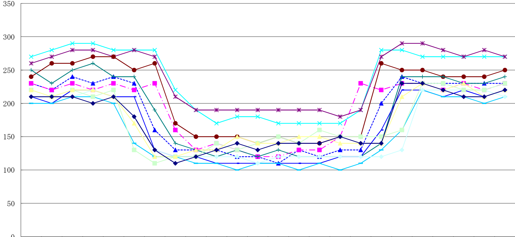
〔使用電力量kWh〕 各月指定日(最大電力量計測日)のロードカーブ(令和4年10月~令和5年9月)(清洲受電所)
