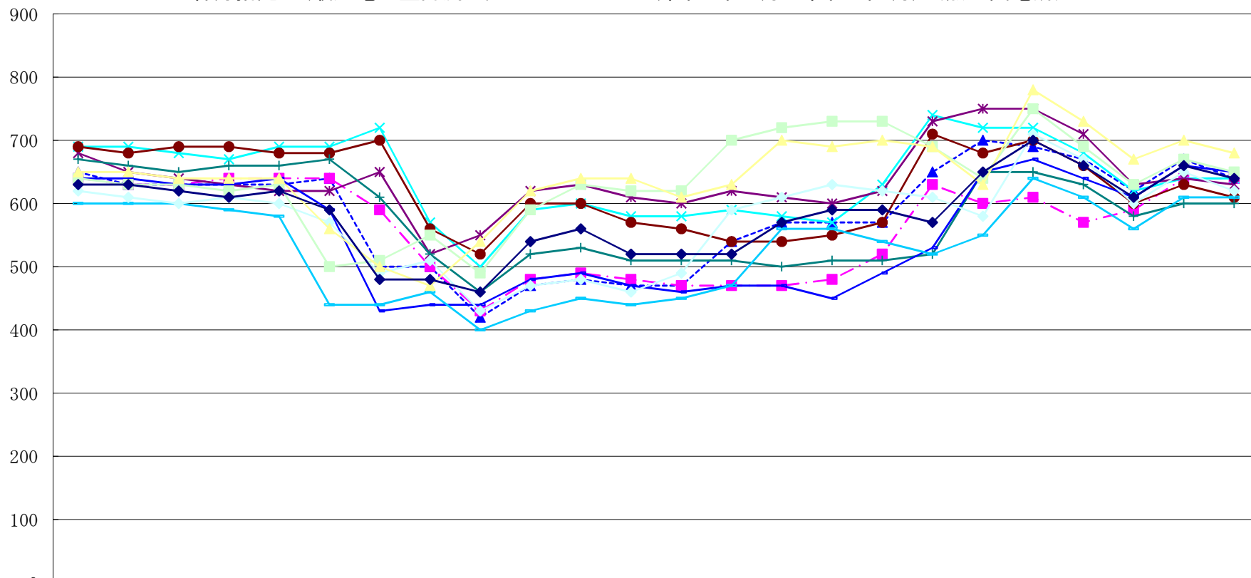
[使用電力量kWh] 各月指定日(最大電力量計測日)のロードカーブ(令和4年10月~令和5年9月)(黒川受電所)
