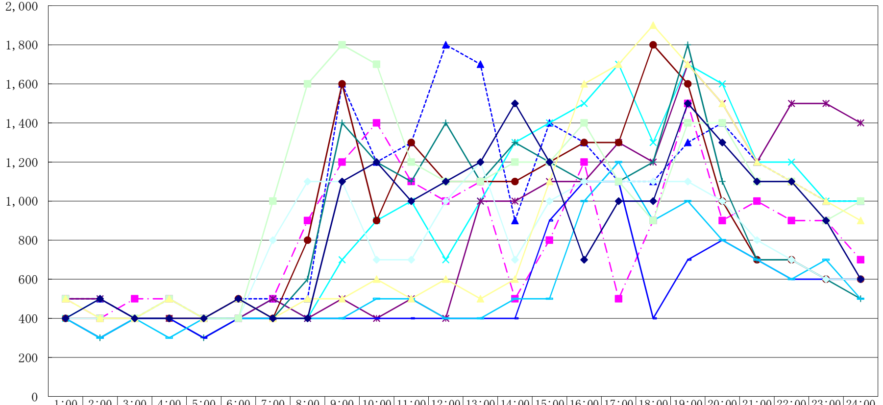
〔使用電力量kWh〕 各月指定日(最大電力量計測日)のロードカーブ(令和4年10月～令和5年9月)(緑橋受電所)
