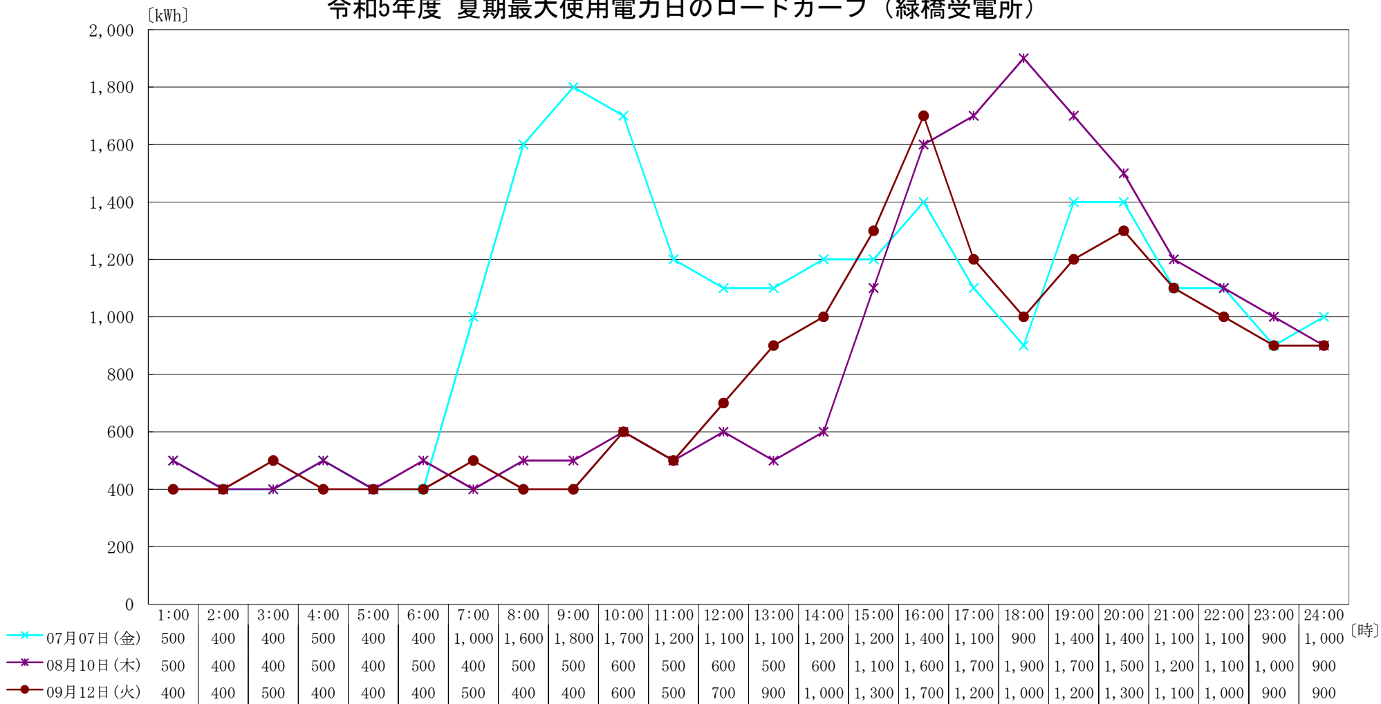
令和5年度 夏期最大使用電力日のロードカーブ (緑橋受電所)
