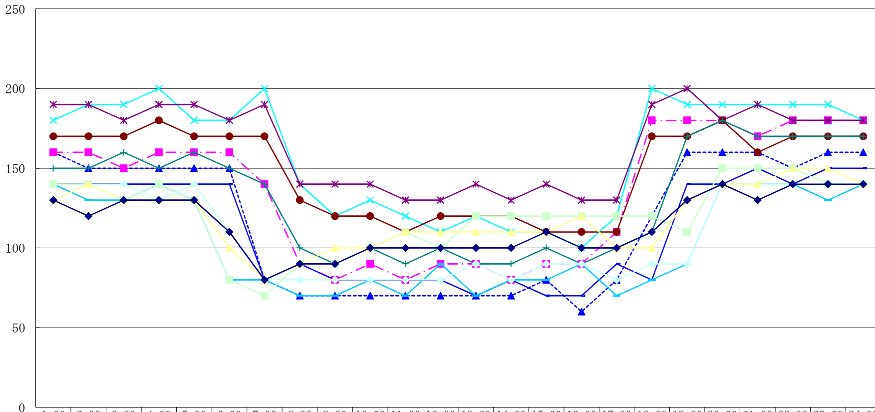
〔使用電力量kWh〕 各月指定日(最大電力量計測日)のロードカーブ(令和4年10月~令和5年9月)(千音寺受電所)
