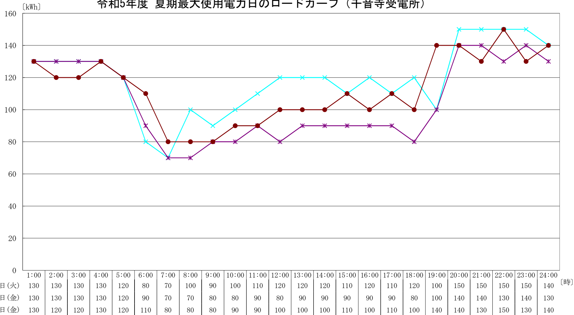
令和5年度 夏期最大使用電力日のロードカーブ (千音寺受電所)
